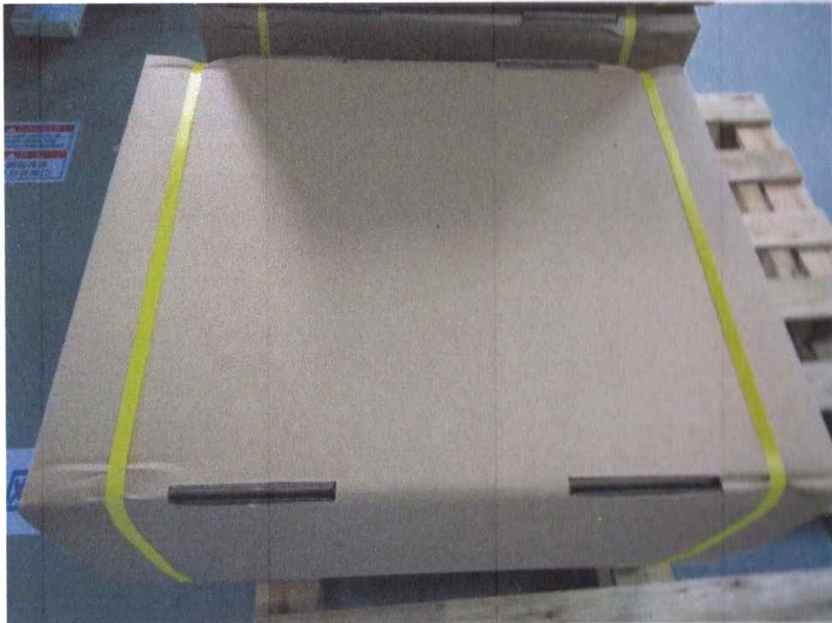
图四, 确认 PA2651 无漏装后, 将 26 的内箱与外箱配合并打包装带待出货
